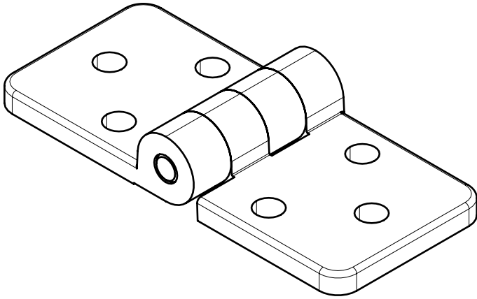
SCALE 1:2
