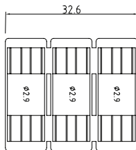
EFA04 71 X01 Ø2.9 Coupler Clip
