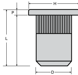
Flachkopf
