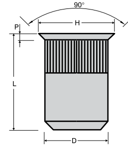
Reduzierter Senkkopf
